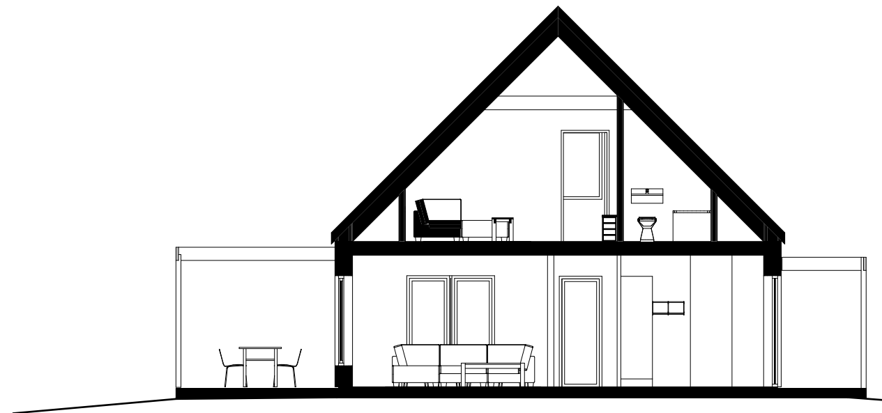
Sektion B-B
