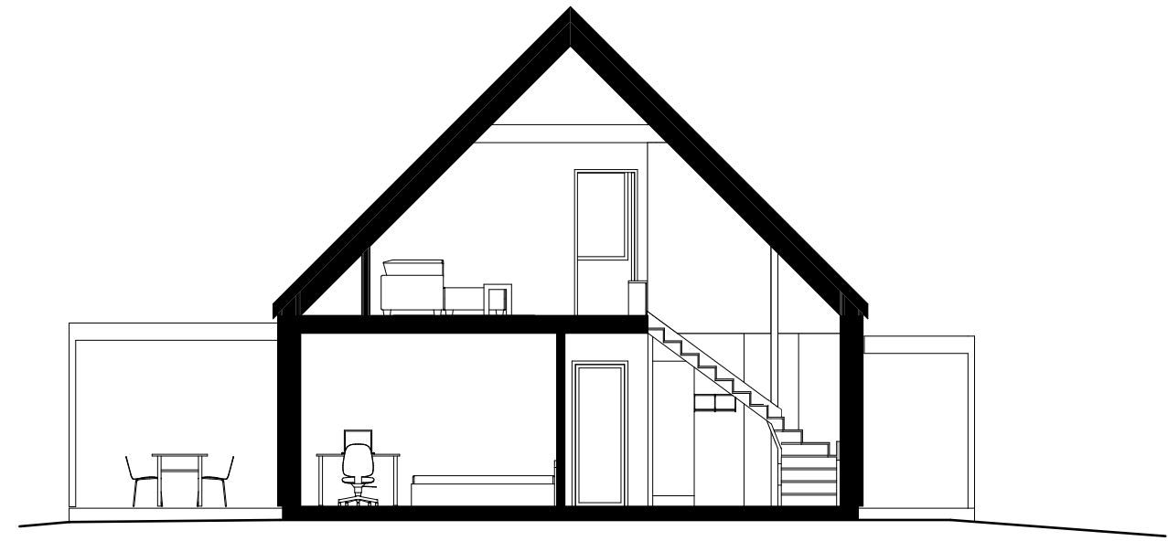
Sektion C-C
